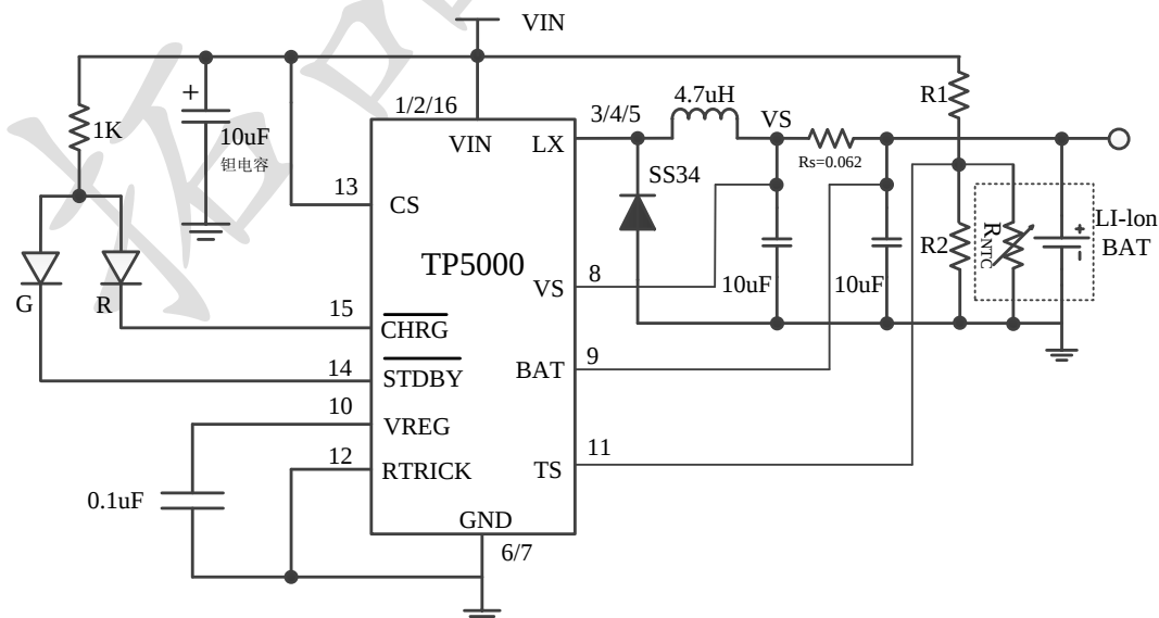
图 1 TP5000 为 4.2V 锂离子电池 1.5A 充电 (150mA 预充) 应用示意图
