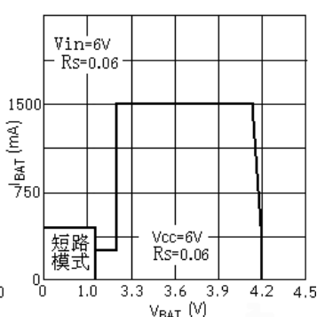
充电电流与电池电压关系
