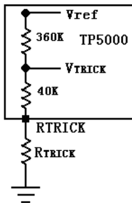
图7 R_{TRICK} 端内部电路图
