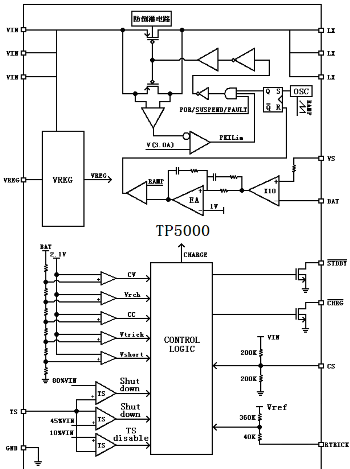
图 3 TP5000 功能框图
